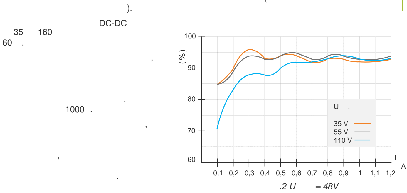
Buck-boost DC-DC
